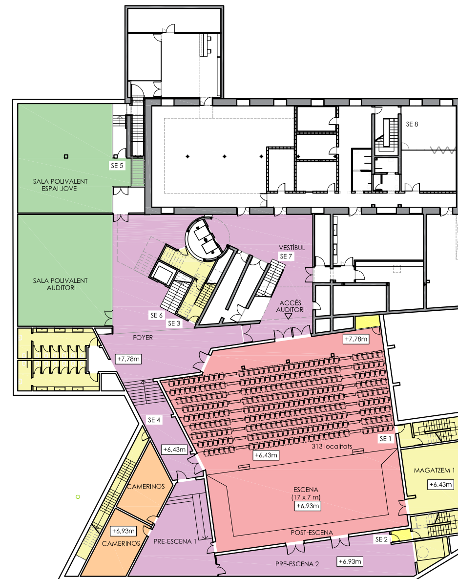
PLANTA SOTERRANI
