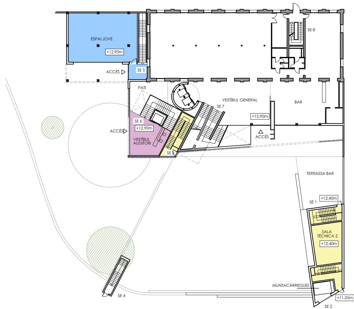
PLANTA BAIXA
