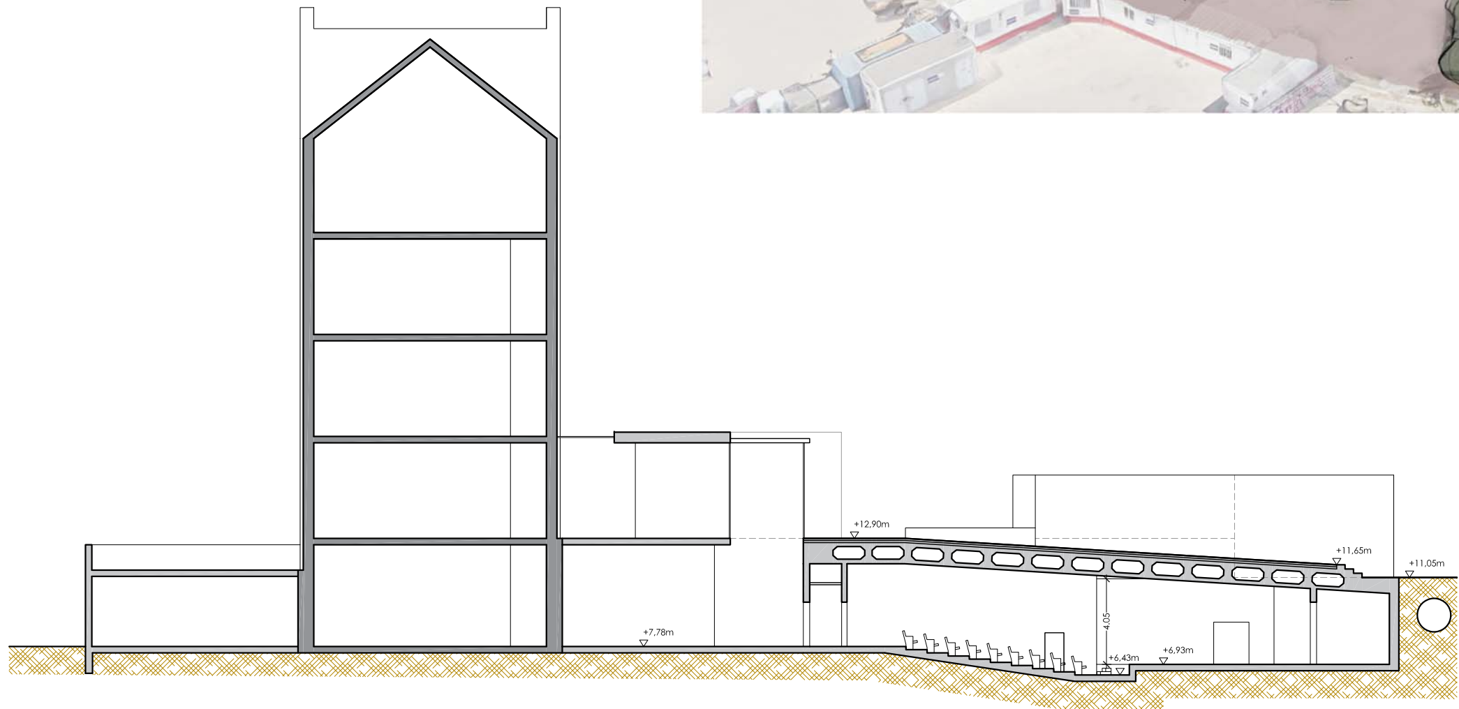
SECCIÓ LONGITUDINAL
