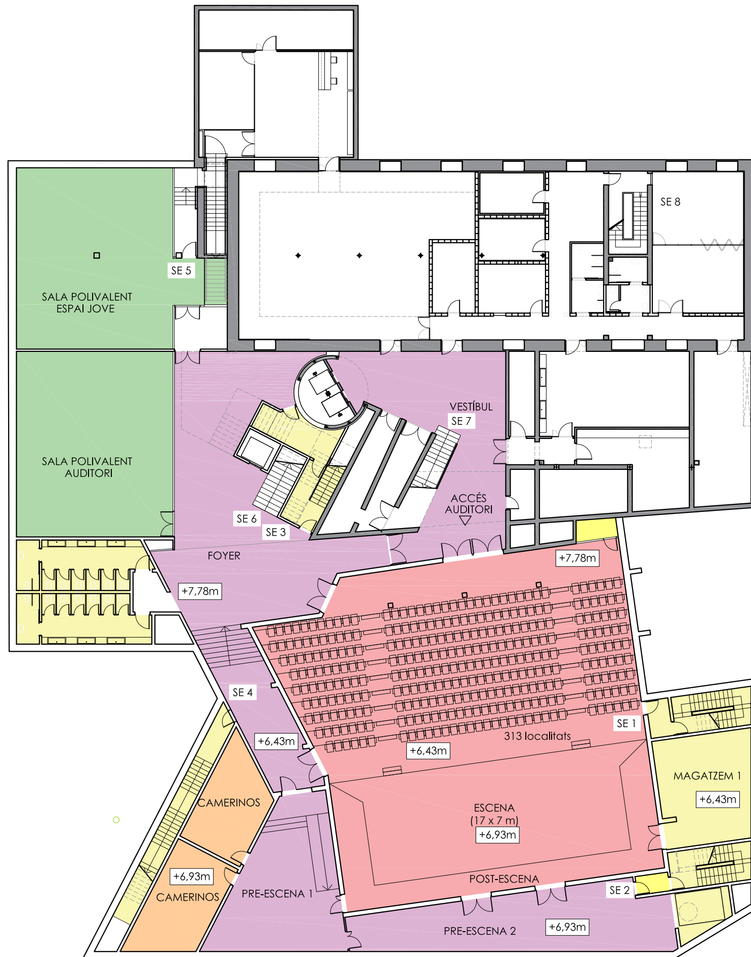
PLANTA SOTERRANI
